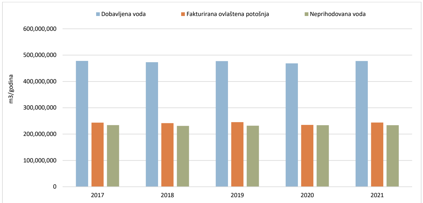
Slika 2.13. Osnovna bilanca vode za razini RH za posljednjih 5 godina (2017.-2021.)
