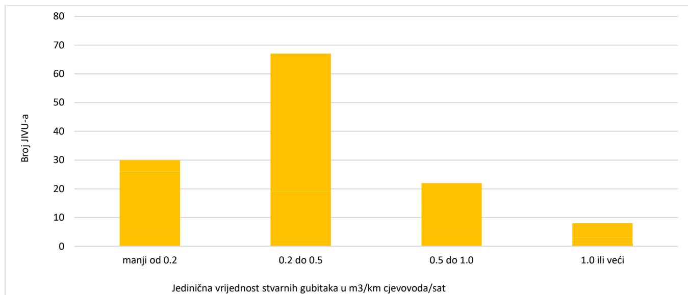
Slika 2.37. Grupiranje vodoopskrbnih sustava u RH prema jediničnoj vrijednosti stvarnih gubitaka u m³/km cjevovoda/sat
