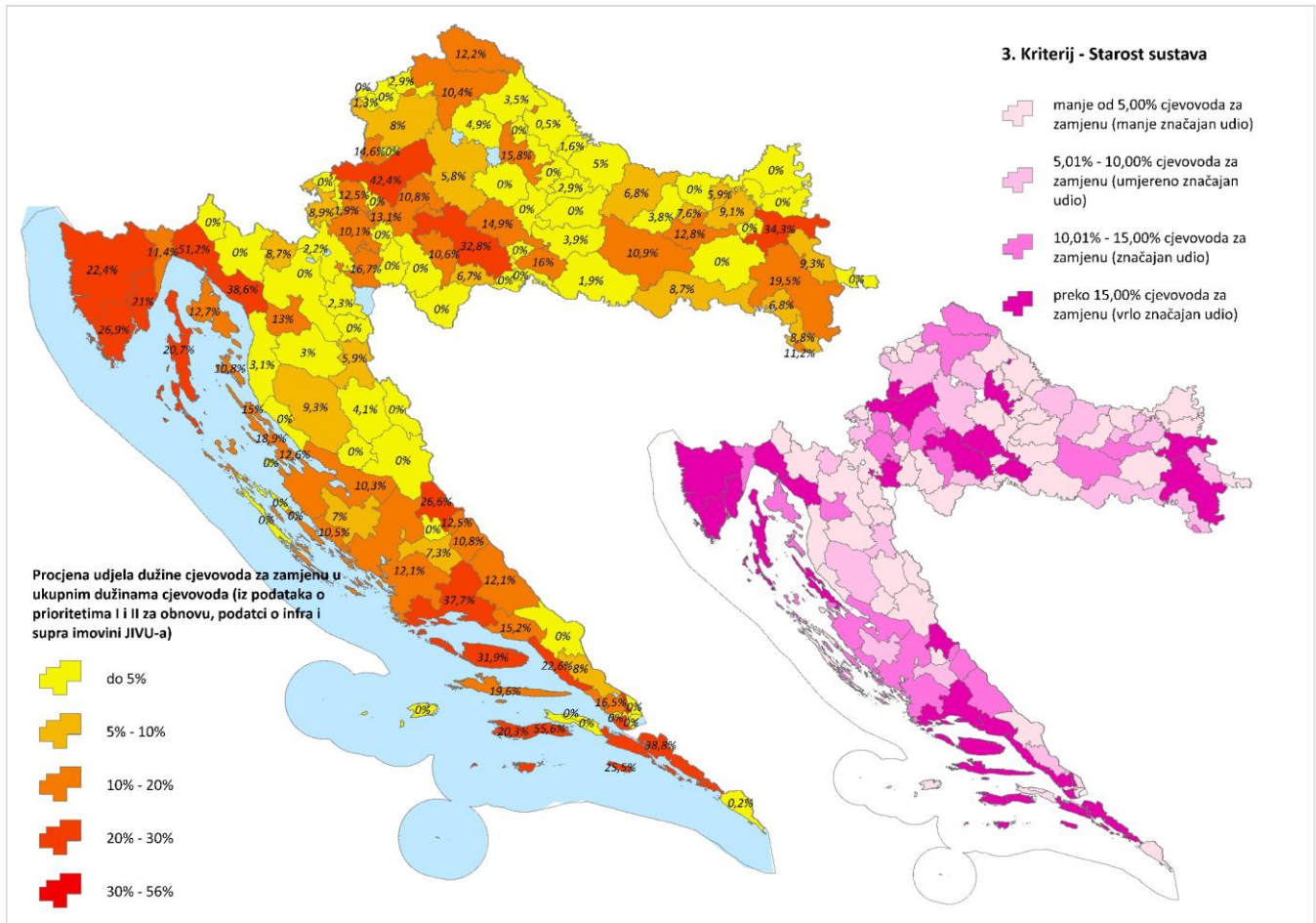
Slika 3.13. Prostorni raspored veličine potrebne obnove cjevovoda u I. i II. prioritetnoj skupini (s prikazom % zamjene, lijevo) i 3. Kriterija (desno)
