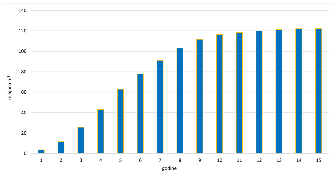
Slika 3.37. Kumulativ učinaka (smanjenje NRW-a, m³)
