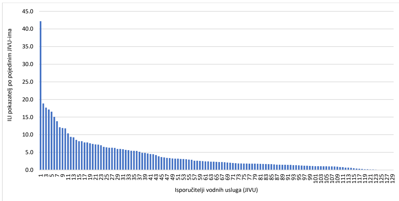
Slika 2.26. Raspodjela vrijednosti ILI pokazatelja po pojedinim JIVU-ima u RH
