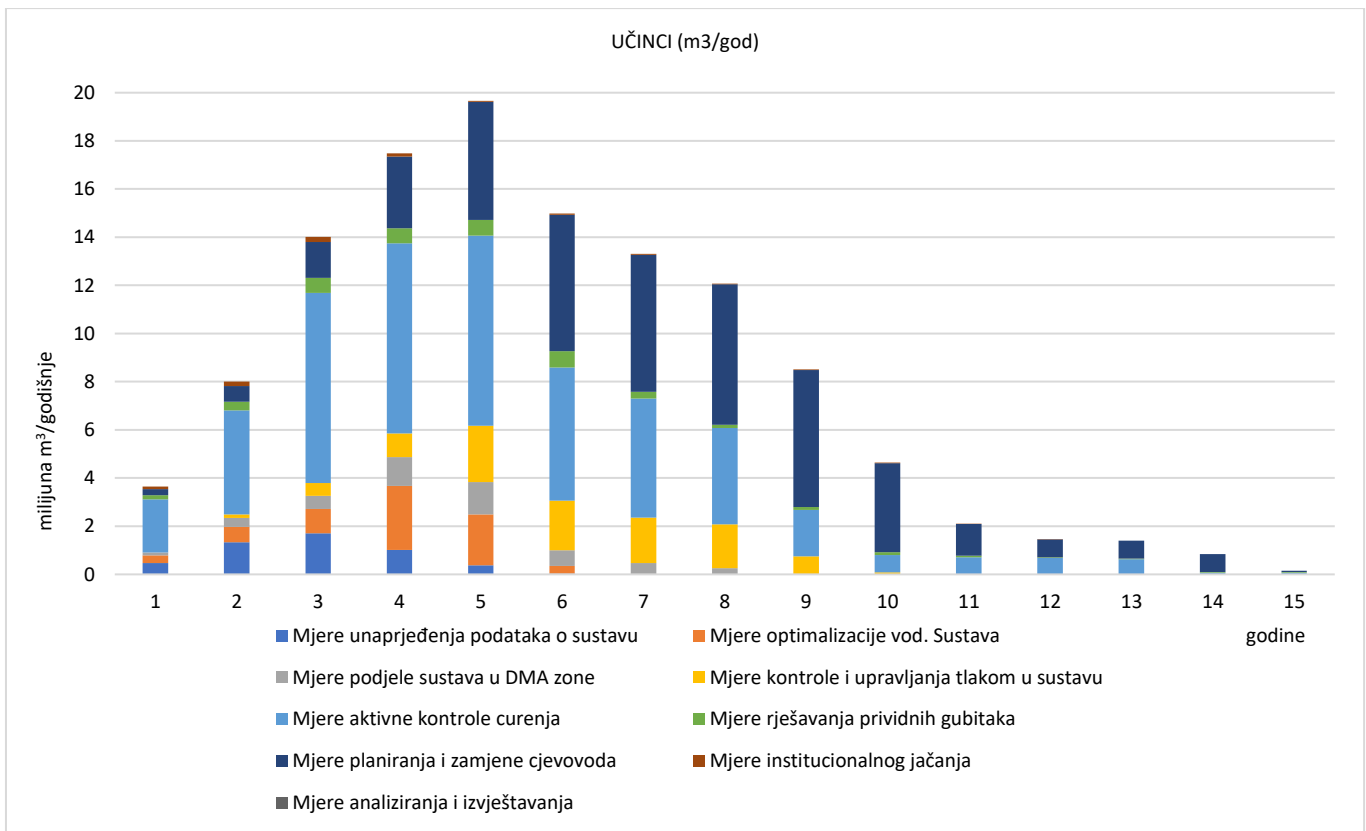
Slika 3.39. Učinci mjera smanjenja gubitaka po godinama (m³/god)
