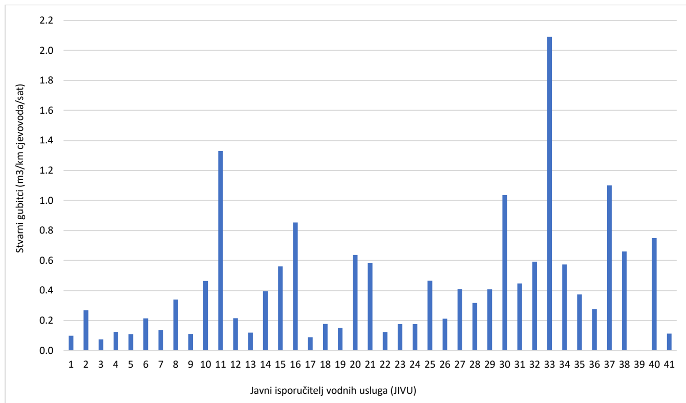
Slika 2.36. Raspodjela jediničnih vrijednosti Stvarnih gubitaka u m³/km cjevovoda/sat, po uslužnim područjima
