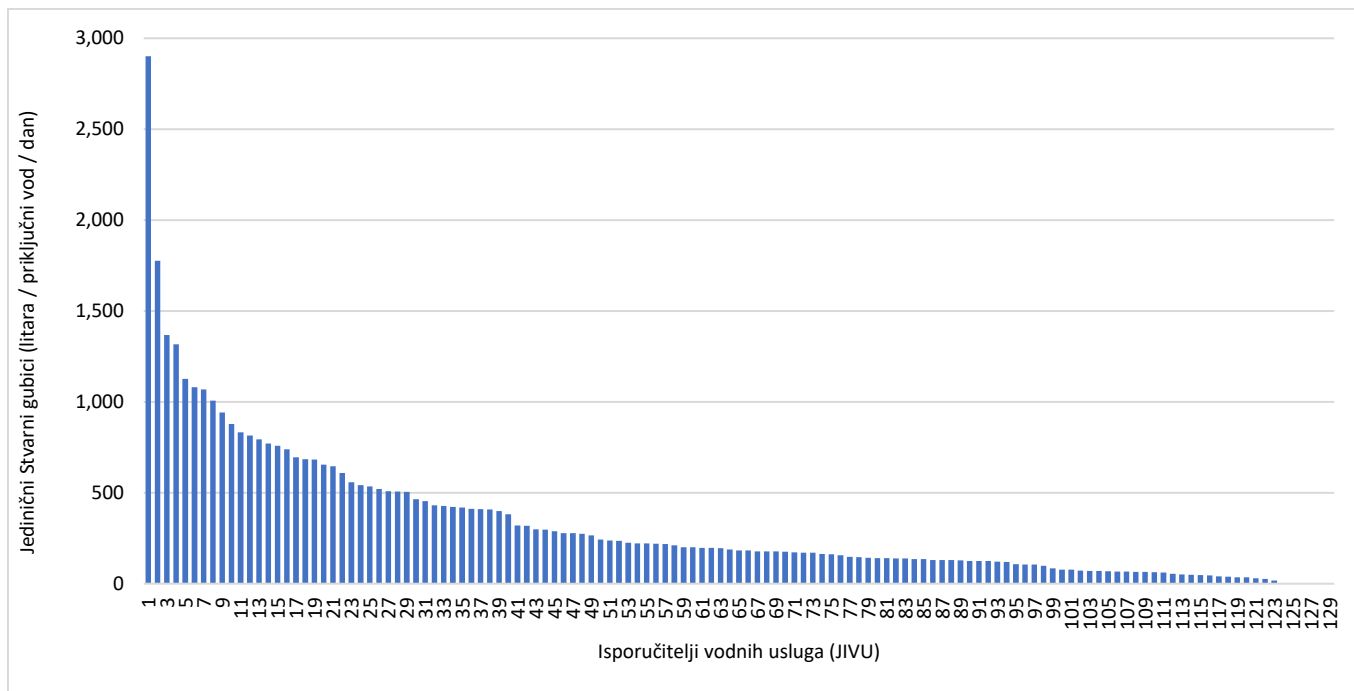
Slika 2.31. Raspodjela jediničnih vrijednosti Stvarnih gubitaka u litara/priključni vod/dan, po pojedinim JIVU-ima
