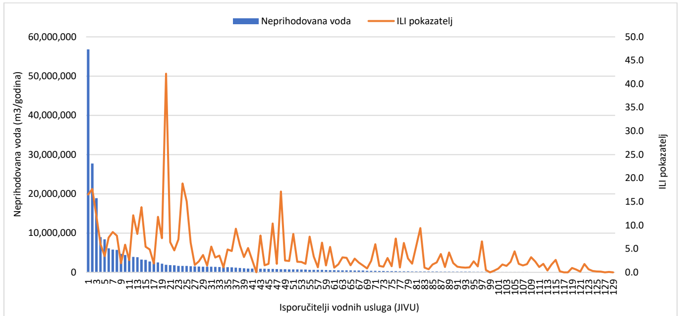
Slika 2.28. Odnos ILI pokazatelja i neprihodovane vode u m 3 /godina po pojedinim JIVU-ima
