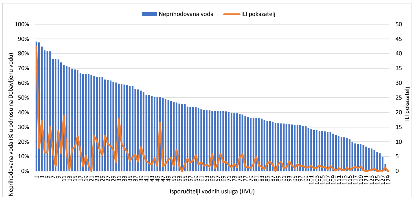
Slika 2.29. Odnos ILI pokazatelja i neprihodovane vode u % po pojedinim JIVU-ima
