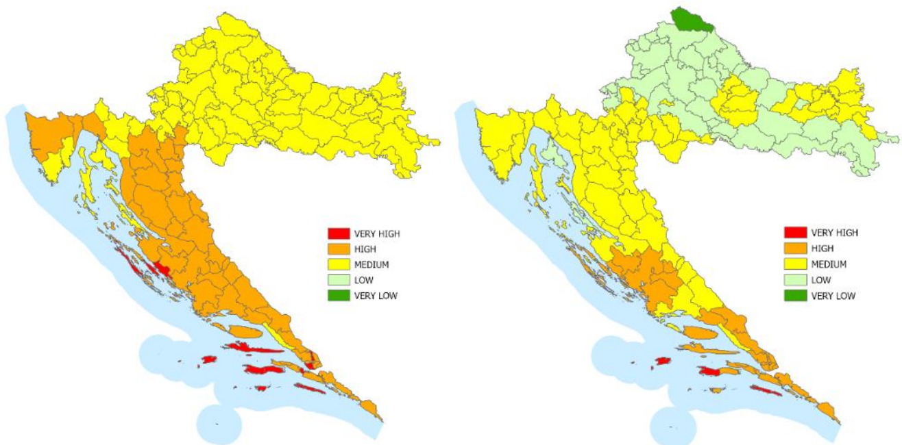
Slika 3.16. Klase ozbiljnosti klimatskih promjena zasnovane na RPC 4.5 (lijevo) i RPC 8.5 (desno) scenarijima (utjecaj temperature uzet u obzir)
